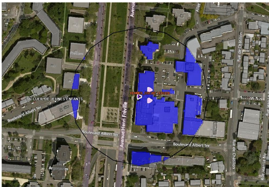
Fond de carte (photo aérienne), source : bing. Logiciel de simulation Cellerity, éditeur Orange Labs
