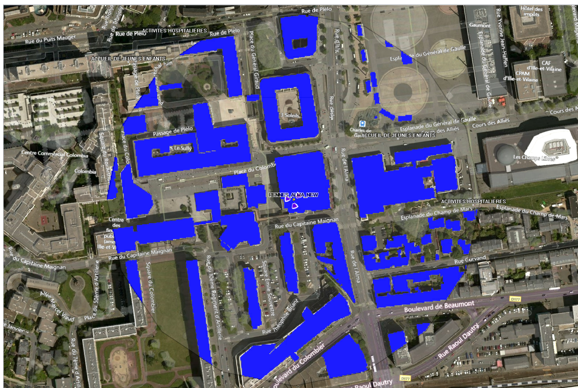
Fond de carte (photo aérienne), source : bing. Logiciel de simulation Cellerity, éditeur Orange Labs
