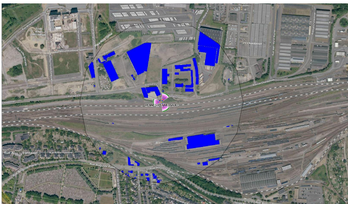
Fond de carte (photo aérienne), source : bing. Logiciel de simulation Cellerity, éditeur Orange Labs
