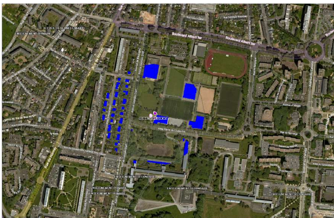
Fond de carte (photo aérienne), source : bing. Logiciel de simulation Cellergy, éditeur Orange Labs
