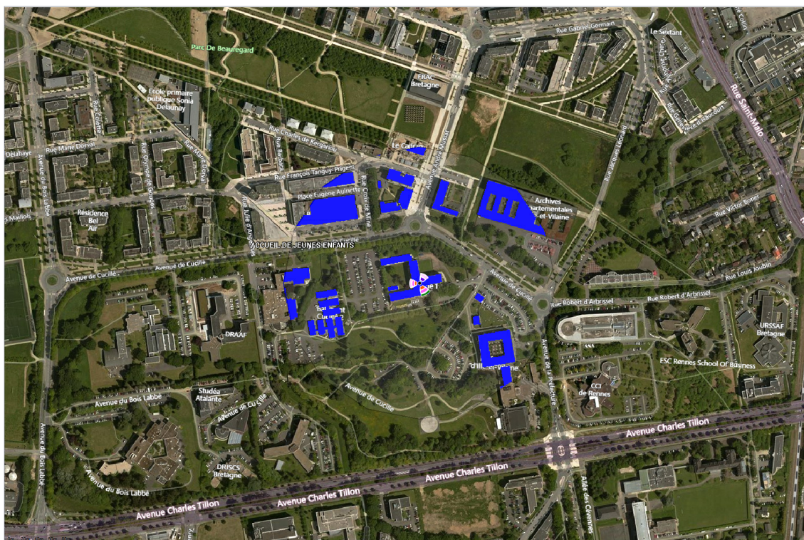
Fond de carte (photo aérienne), source : bing. Logiciel de simulation Cellergy, éditeur Orange Labs
